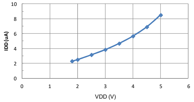
静态电流 vs. 工作电压
